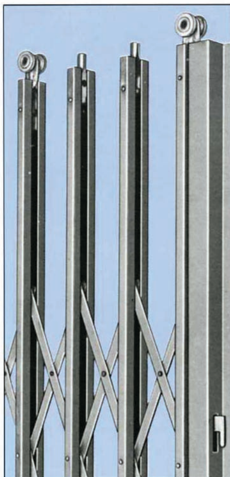
Supporto a carrello portante con cuscinetti a sfera e ometti di guida
